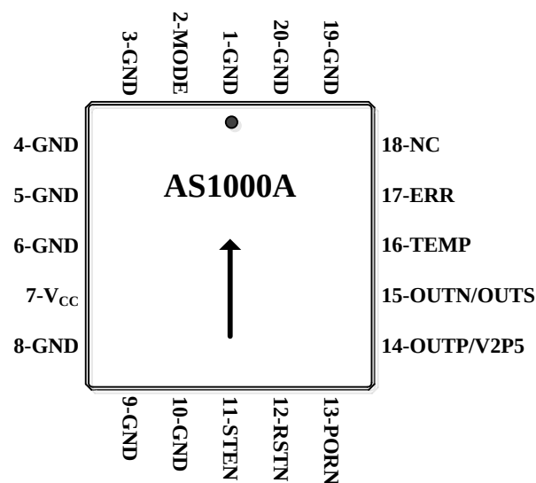
图 1. AS1000A 引脚排布图（顶视）
