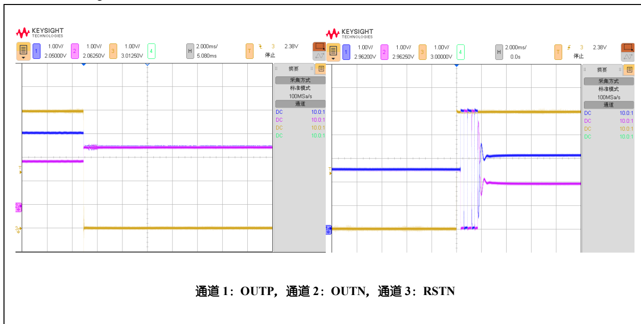
图 4. 复位拉低、拉高时输出波形曲线
