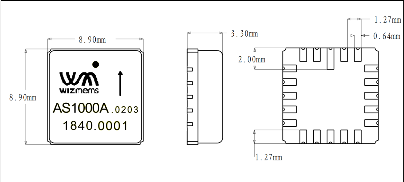
图 6. AS1000A 封装 (LCC20) 外形尺寸图
